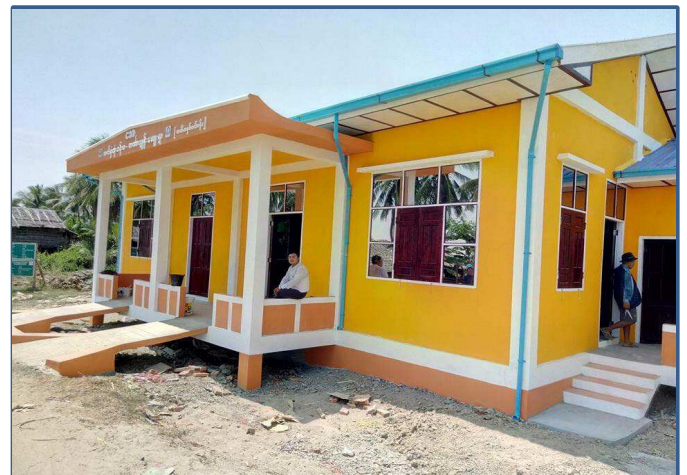
ချောင်းဆုံမြို့နယ် ဟင်္သာကျွန်းကျေးရွာ ကျေးရွာစာကြည့်တိုက်တည်ဆောက်ခြင်း
