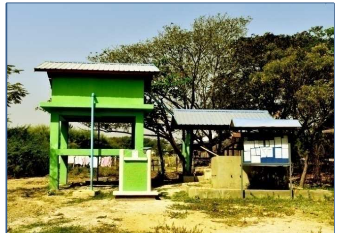
ပျော်ဘွယ်မြို့နယ် ရုံးပင်ကန်ကျေးရွာ ရေစင်၊ရေပိုက်သွယ်တန်းခြင်း
